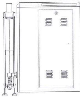
左视图
